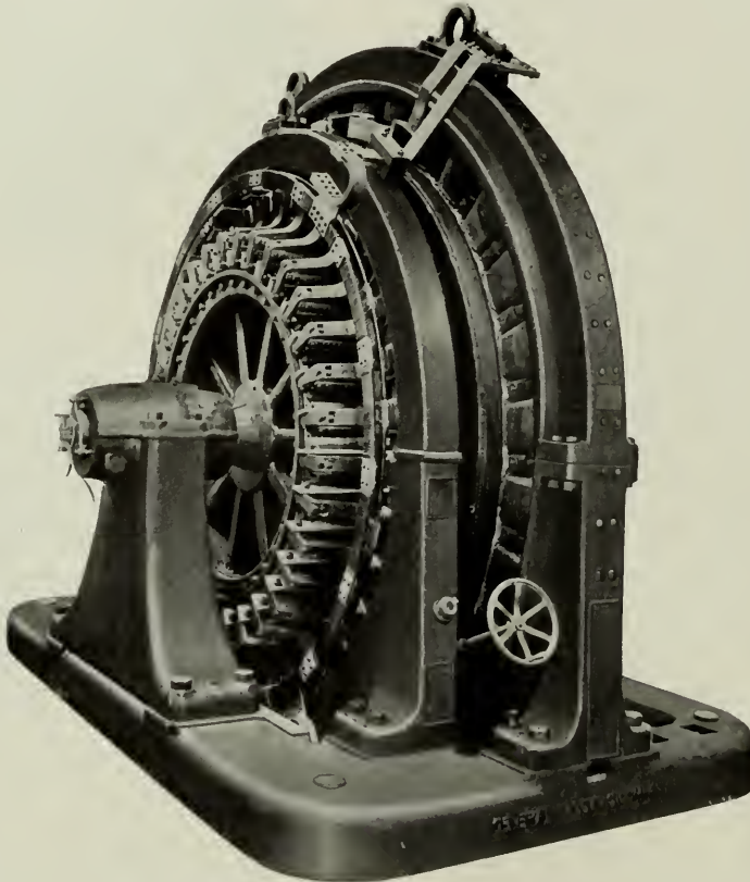
Fig. 27. 580-kw. 225-r.p.m. 580-volt Synchronous Converter
