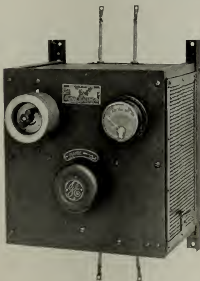
Fig. 8. Six-ampere, 75-volt Rectifier
