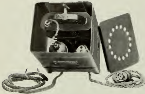
Fig. 39. 2-amp. 7.5-volt Tungar Rectifier
